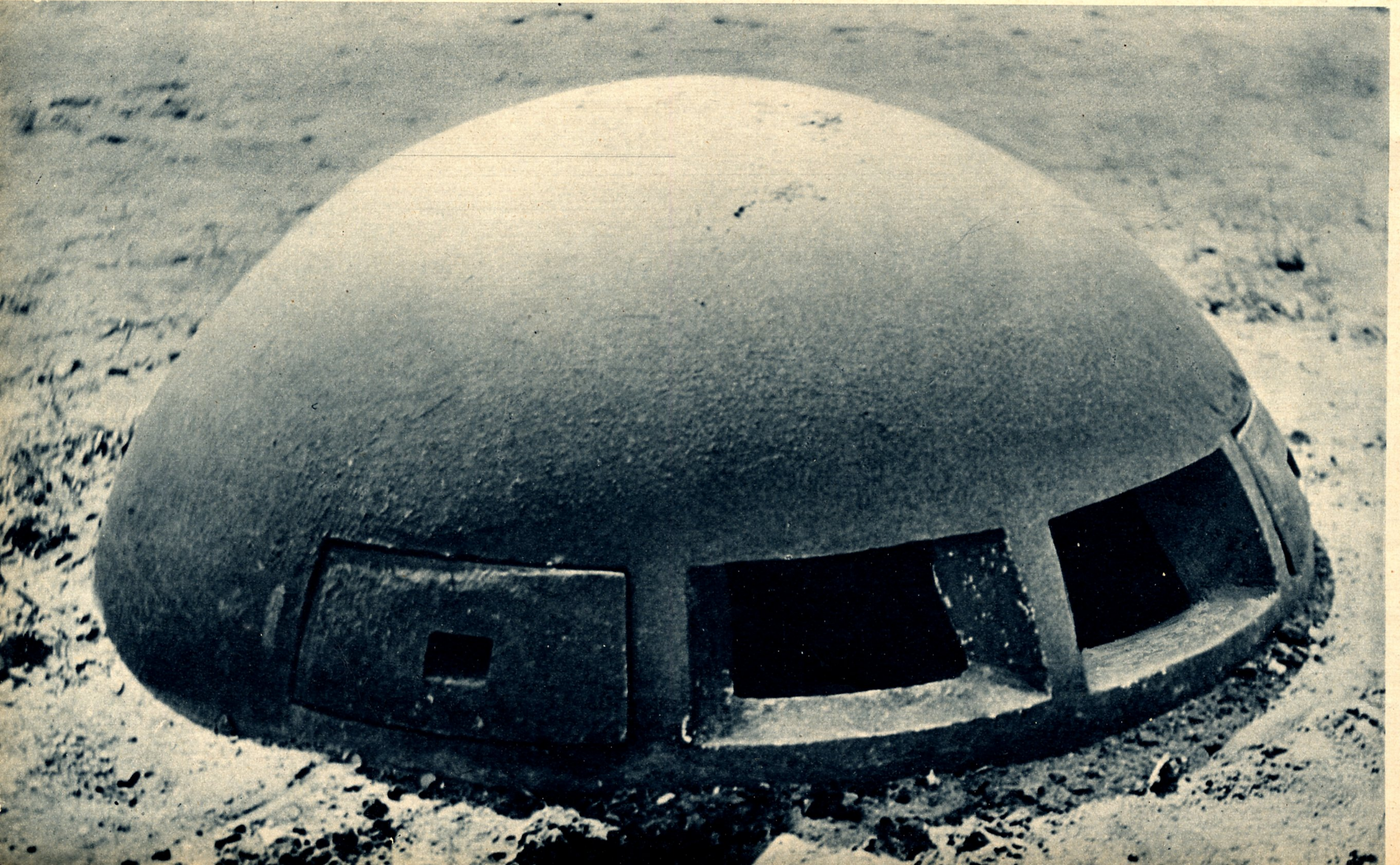
Unten: Diese Panzerkuppel eines Beobachtungsstandes ist das Auge eines großen Unterkunfts- und Kampfwerkes, das tief unter ihm in den Berg eingebaut ist
